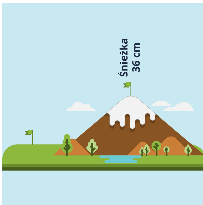
Grubość pokrywy śnieżnej Piątek 16.05.2025 08:00
