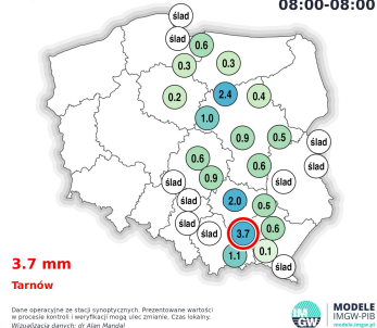
Suma opadu Czwartek / Pt. 15.05.25 / 16.05.25 08:00-08:00
