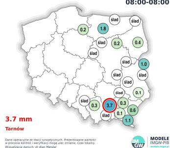
Suma opadu Wtorek / Śr. 13.05.25 / 14.05.25 08:00-08:00
