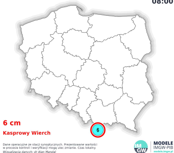
Grubość pokrywy śnieżnej Piątek 16.05.2025 08:00
