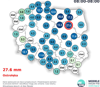
Suma opadu Niedziela / Pon. 18.05.25 / 19.05.25 08:00-08:00
