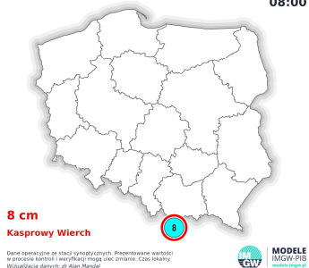
Grubość pokrywy śnieżnej Czwartek 15.05.2025 08:00
