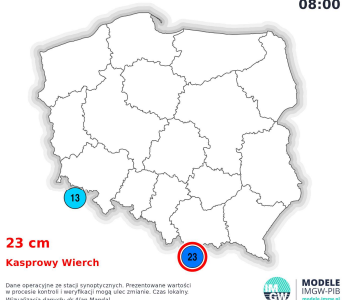
Grubość pokrywy śnieżnej Wtorek 20.05.2025 08:00
