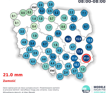
Suma opadu Piątek / Sob. 16.05.25 / 17.05.25 08:00-08:00
