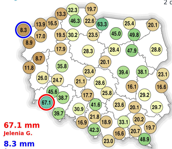
Suma opadu Niedziela / Pon. 18.05.25 / 19.05.25 08:00-08:00
