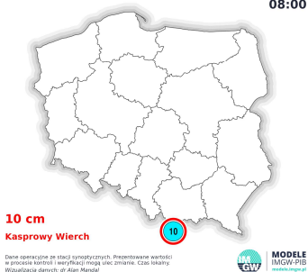
Grubość pokrywy śnieżnej Środa 14.05.2025 08:00
