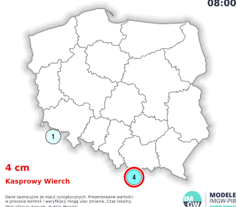
Grubość pokrywy śnieżnej Sobota 17.05.2025 08:00
