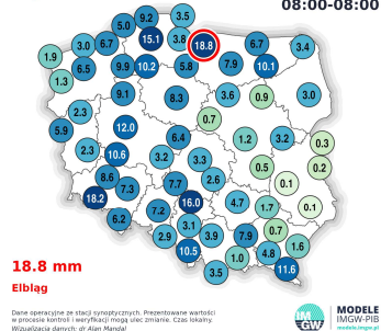
Suma opadu Poniedziałek / Wt. 19.05.25 / 20.05.25 08:00-08:00
