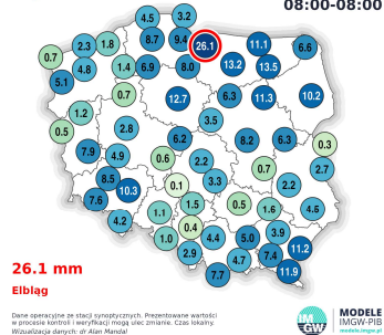
Suma opadu Sobota / Niedz. 17.05.25 / 18.05.25 08:00-08:00
