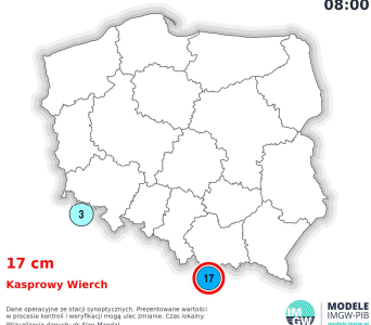
Grubość pokrywy śnieżnej Niedziela 18.05.2025 08:00
