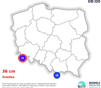
Grubość pokrywy śnieżnej Poniedziałek 19.05.2025 08:00
