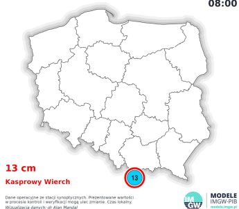
Grubość pokrywy śnieżnej Wtorek 13.05.2025 08:00
