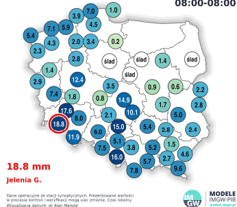
Suma opadu Wtorek / Śr. 20.05.25 / 21.05.25 08:00-08:00
